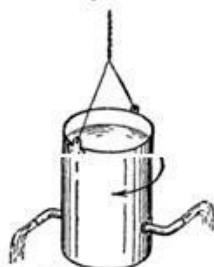
Рис. 320. Ведрко вращается в сторону, обратную направлению вытекания струи
