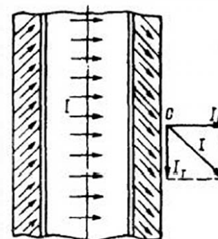
Рис. 46. Принципиальная схема импульсного униполярного генератора с самовозбуждением I_H — нормальная составляющая тока; I_T — тангенциальная составляющая
