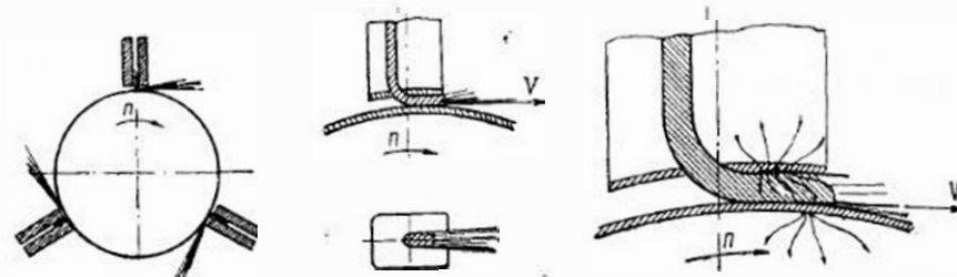
Рис. 35. Эскиз струевого токосъемного устройства
