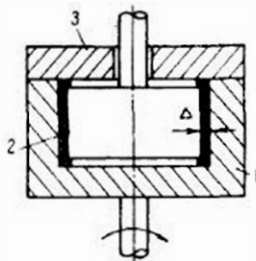
Рис. 37. Устройство для определения механических потерь трения жидкости
