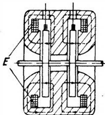
Рис. 13. Дискосая униполярная машина Форбса
