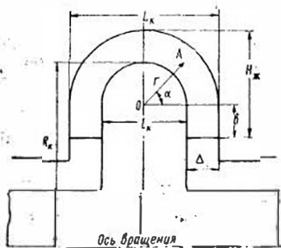
Рис. 66. Кольцевой контакт с плавными очертаниями токо-съемных электродов
