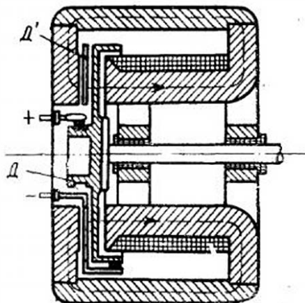
Рис. 14. Униполярная машина Тюрн с компенсационным диском
