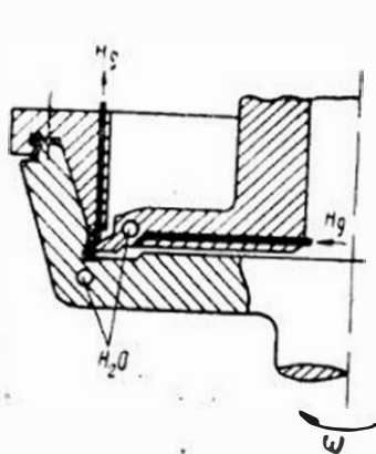
Рис. 32. Поперечный разрез униполярной машины с внешним ротором
