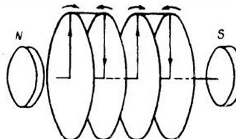
Рис. 12. Способ соединения дисков для сложения индуктированных в них э. д. с.
