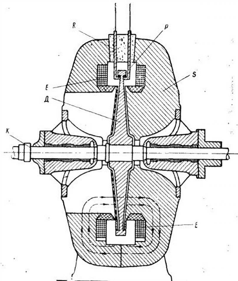
Рис. 15. Униполярный генератор Б. Угримова с дисковым ротором ( D ) и ртутным контактом ( P )
