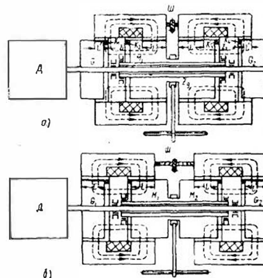
Рис. 51. Продольный разрез униполярного преобразователя вращающего момента
