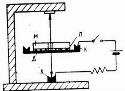
Рис. 7. Экспериментальная дисковая модель Дас Гупта
