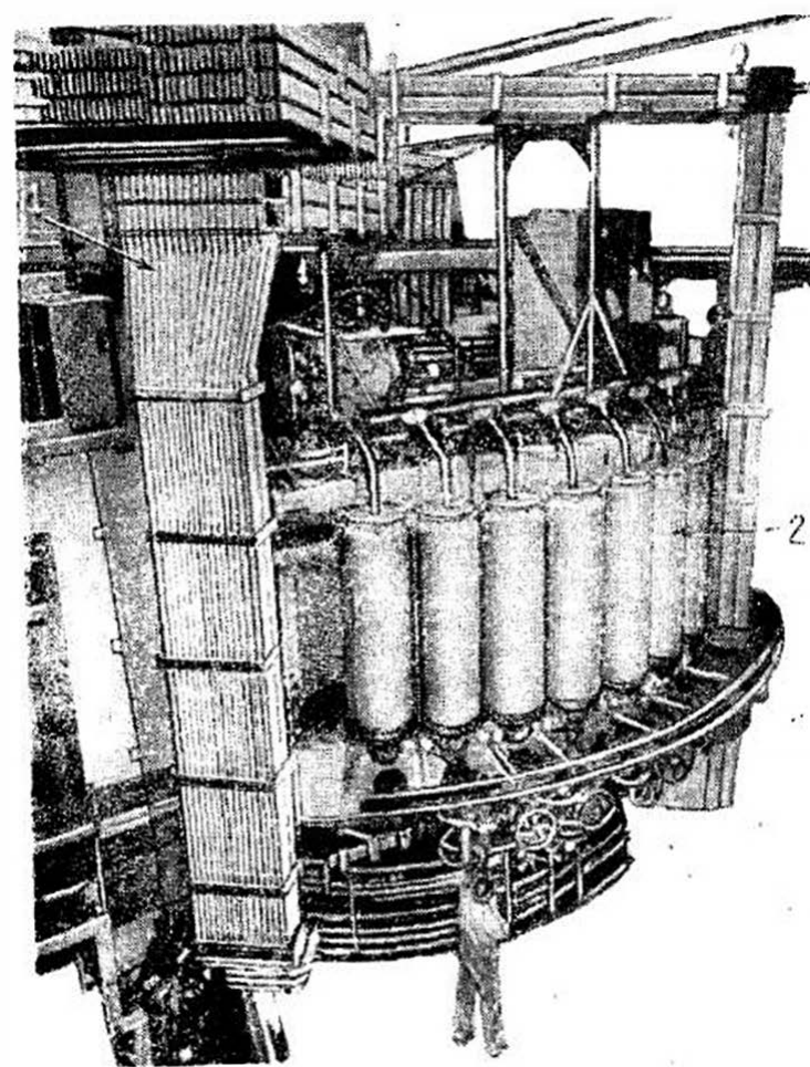
Рис. 4. Внешний вид импульсного униполярного генератора Австралийского национального университета 1 — шинный провод, 2 — блин со сплавом NaK
