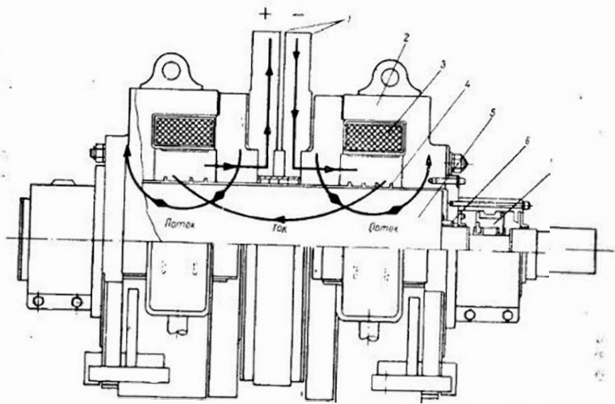
Рис. 48. Продольный разрез импульсного униполярного генератора фирмы Allis Chalmers на 300 ка
