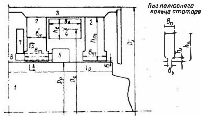
Рис. 80. Конструктивная схема униполярной машины с цилиндрическим ротором
