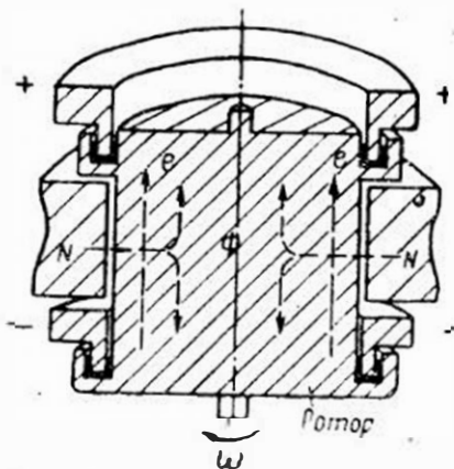
Рис. 33. Токосъемные устройства в униполярной машине с вертикальной осью вращения
