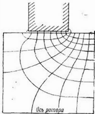
Рис. 60. Картина магнитного поля
