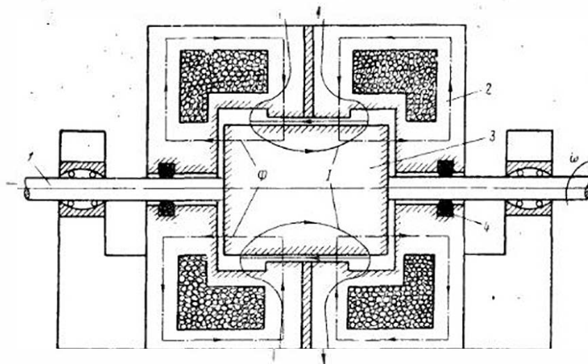
Рис. 43. Принципиальная схема униполярной машины Пулэна
