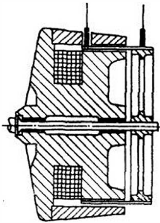
Рис. 17. Униполярный генератор Перу с колоколообразным ротором
