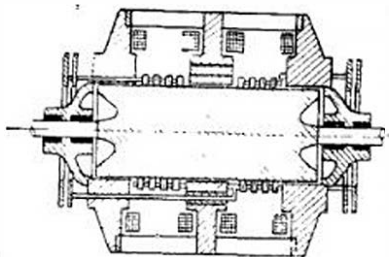
Рис. 24. Продольный разрез униполярной машины Сомеда
