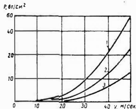
Рис. 38. Зависимость удельных потерь трения ртути от линейной скорости поверхности и толщины слоя жидкости
