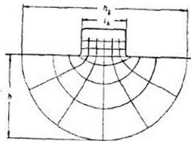
Рис. 75. Растекание тока в стали ротора у основания токоъемного кольца
