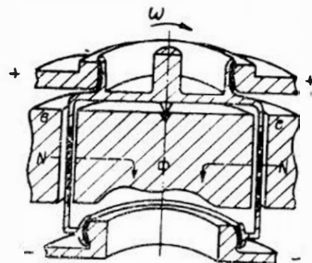
Рис. 34. Поперечный разрез униполярной машины с кольцевыми контактами
