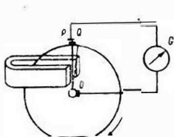
Рис. 5. Схема дисковой модели униполярной машины
