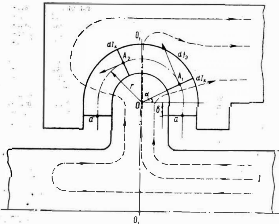
Рис. 78. Протекание тока через токосъемное устройство
