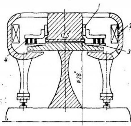
Рис. 18. Униполярный генератор мощностью 90 кВт с Т-образным сечением ротора 1 — токосъемное кольцо; 2 — обмотка возбуждения; 3 — контактное кольцо; 4 — щетки
