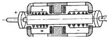
Рис. 22. Униполярный генератор Пуарсона на ток 15 ка
