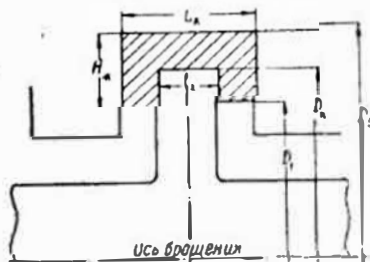
Рис. 65. Кольцевой контакт с П-образным поперечным сечением
