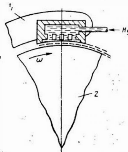
Рис. 36. Эскиз струевого токосъемного устройства 1 — статор; 2 — ротор
