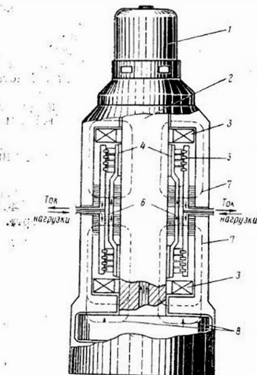
Рис. 27. Униполярный генератор с вертикальным цилиндрическим ротором
