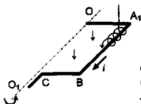
Рис. 14. Точка A_1 активного участка полу контура сблизилась с краем потока на критическое расстояние и первая силовая линия потока завернула на проводник
