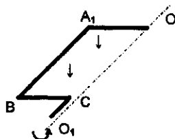
Рис. 15. Полу контур завершил прохождение северной части межполюсного пространства и снова вышел на начальное положение, повернувшись на угол \pi
