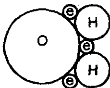
Рис. 3. Положительная молекула воды (три электрона связи)
