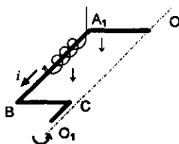
Рис. 16. Начало вхождения полу контура в южную часть межполюсного пространства. Вновь точка A_1 первой вступает во взаимодействие с потоком
