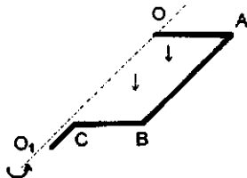
Рис. 12. Полу контур в начальном положении. Его плоскость нормальна к потоку
