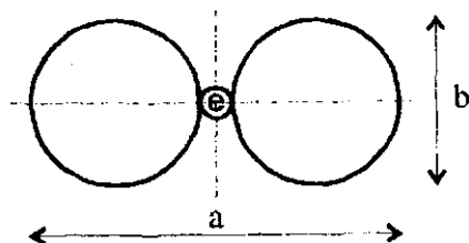
Рис. 1. Одномостиковое соединение пары атомов в молекуле O_2 . a — большая, b — малая оси молекулы
