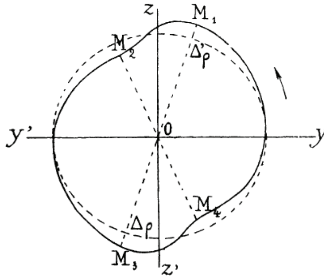
FIGURE 9. Oscillations entretenues par une lampe trois électrodes, d'après Blondel [19, p. 157]
