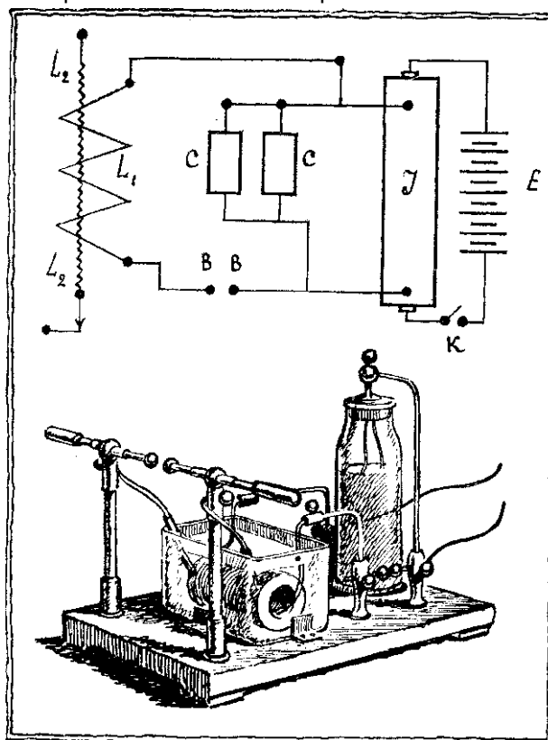
Резонанс-трансформатор Теслы: Е — батарея или другой источник тока. J — индукционная катушка. ВВ — искровой разрядник. СС — батарея лейденских банок. L 1 — первичная катушка трансформатора. L 2 — вторичная катушка трансформатора, К — механический прерыватель. На нижнем рисунке катушки L 1 и L 2 погружены в масло.
