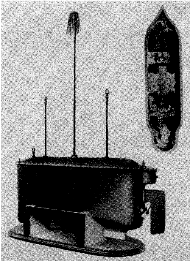
Управляемое по радио судно Николы Теслы, плававшее в бассейне Медисон-сквер-гарден (хранится в музее Теслы в Белграде)
