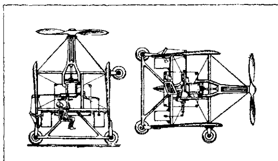
Проект геликоптера Николы Теслы.
