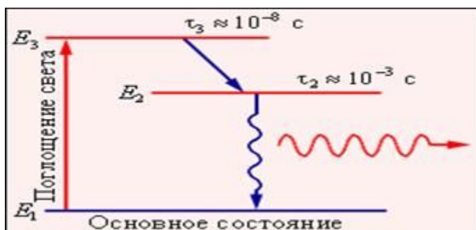
Рисунок 4. Схема рубинового лазера [5].
