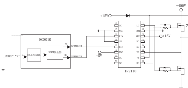
图 8.4b EG8010 正极性 PWM 驱动 IR2110
