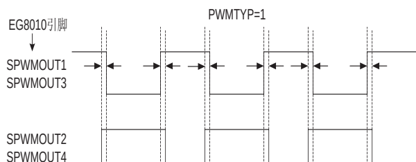
图 8.4c EG8010 负极性 PWM 类型输出
