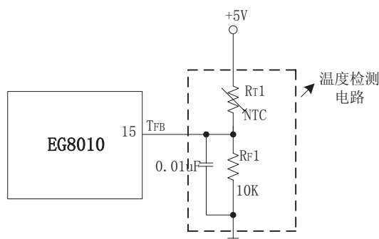
图 8.3a EG8010 温度检测电路
