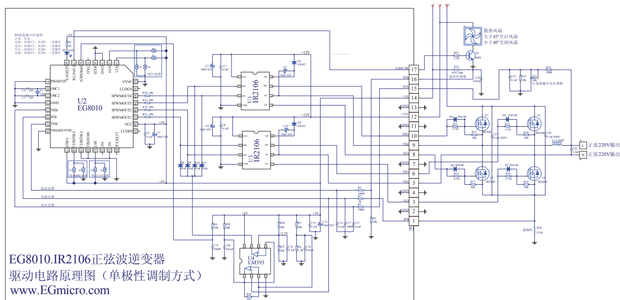
图 6-3. EG8010+IR2106S 纯正弦波逆变器典型应用电路图 (单极性调制方式)
