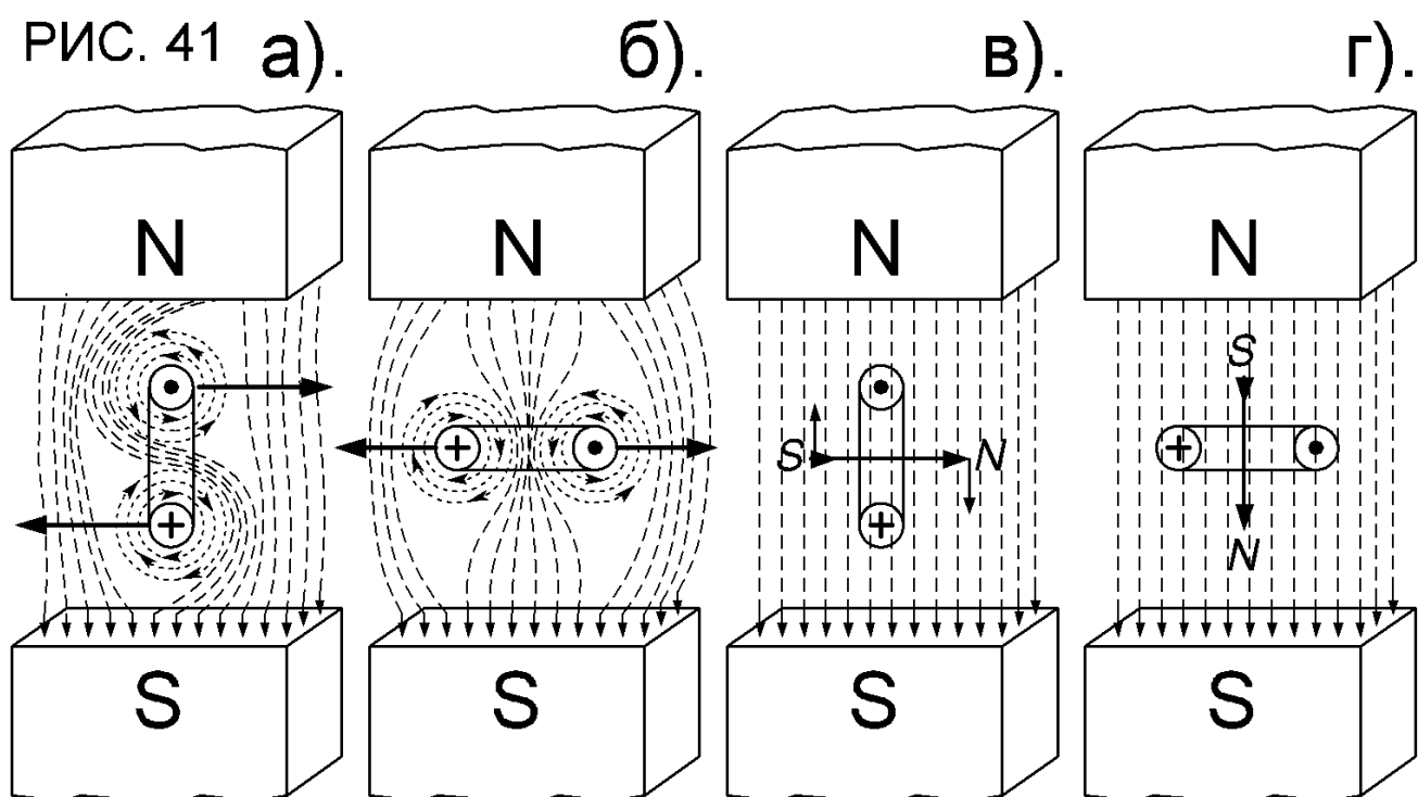
Виток с током в «магнитном» поле.
