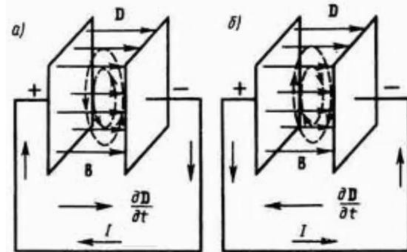
Ток смещения. По Максвеллу
