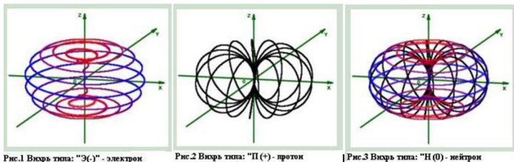
Рис.1 Вихрь типа: "Э(-)" - электрон
