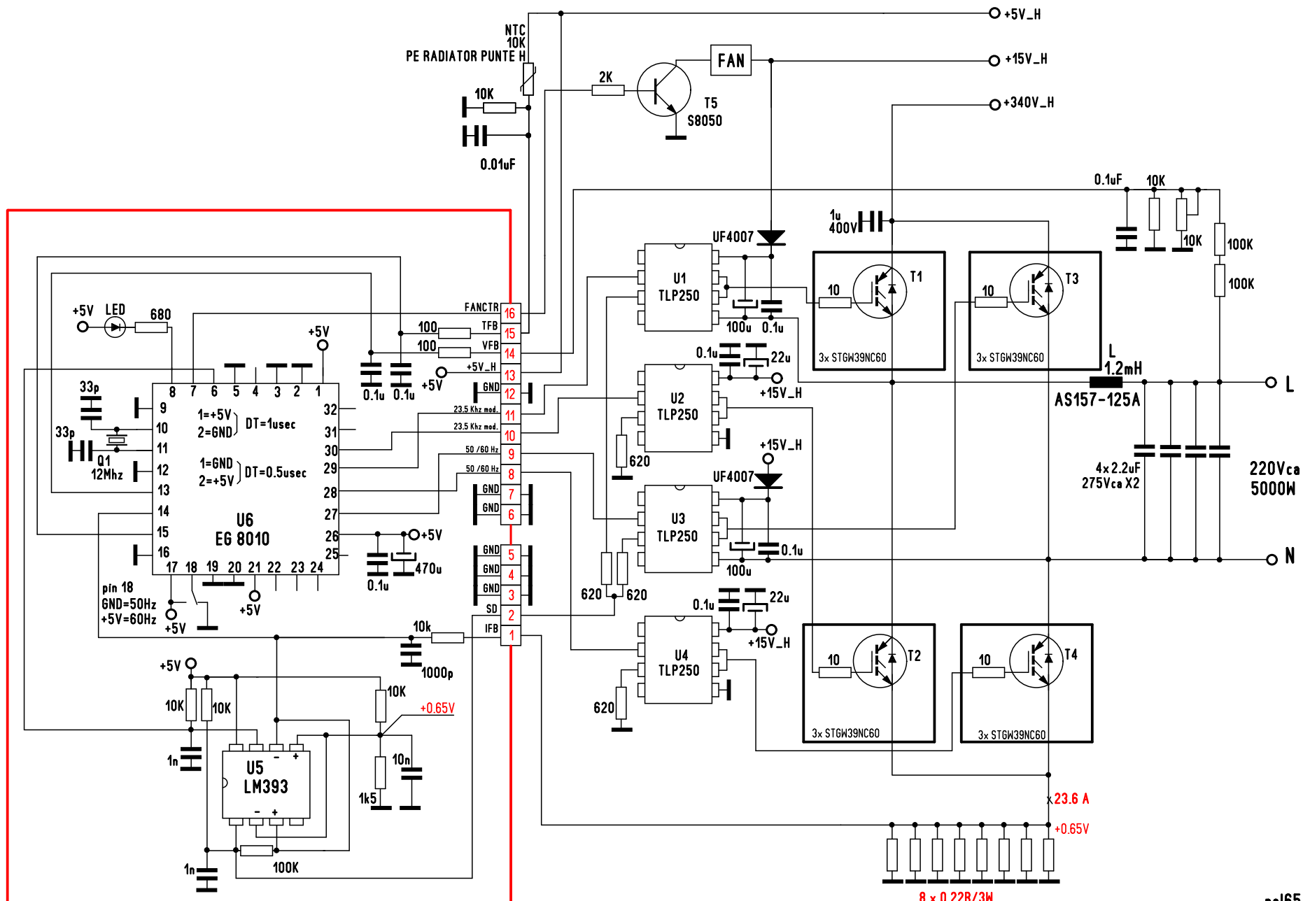
4.Schema puntea H_EG 8010
